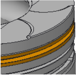
Ni Resist groove insert
